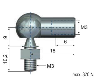
2-M3 Winkelgelenk • Angle joint Joint à angle • Snodo angolare Charnela articulada
