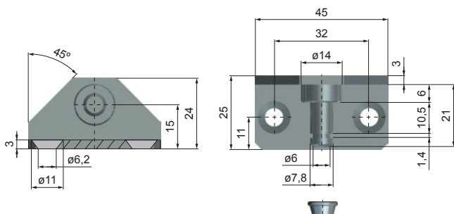
21-VA (für / for 1-M8-VA, 4-M8-VA)
